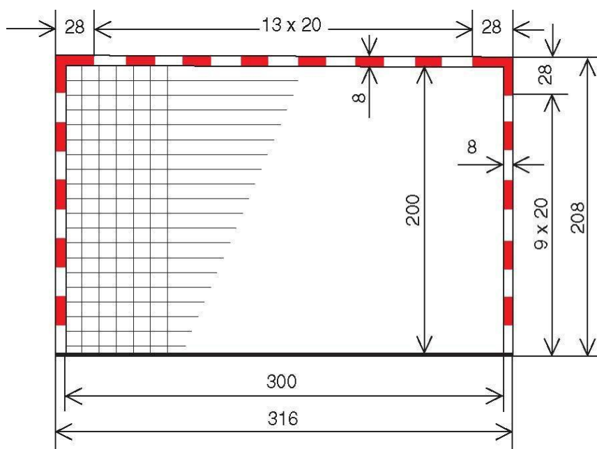
Abbildung 2a: Das Tor
