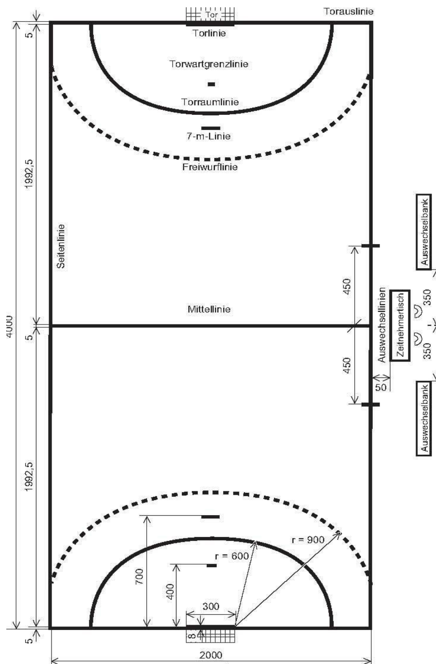
Abbildung 1: Die Spielfläche Alle Maße sind in cm angegeben.
